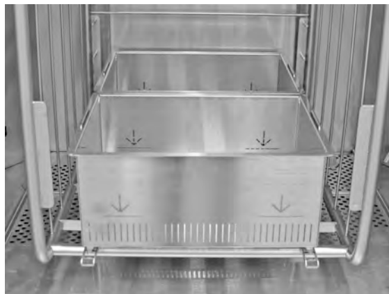
Figure 20 Съдове за събиране на гранули в машината
