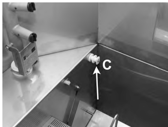
Bild 26 Nivåvakt
