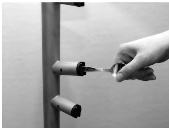
Bild 23 Rengöring av spraymunstycket
