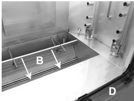
Bild 25 Granulsil och droppspår
