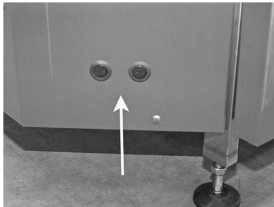
Bild 18 Åtkomst till överhettningsskydden
