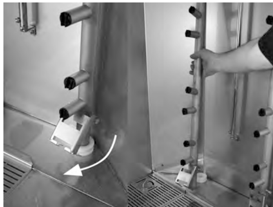
Bild 22 Ta bort sprayröret
