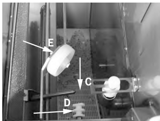
изображение 36 Нижнее сито, датчик уровня и ролики
