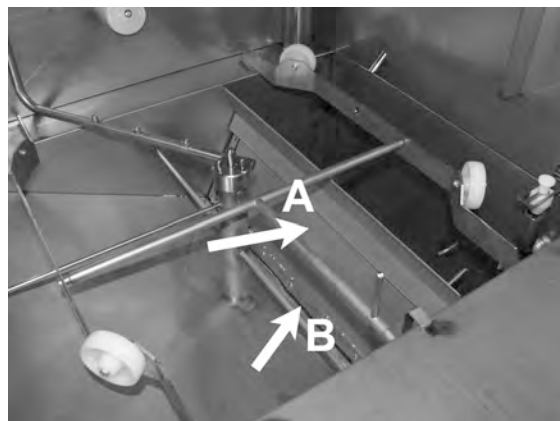
изображение 35 Задвижка гранул
