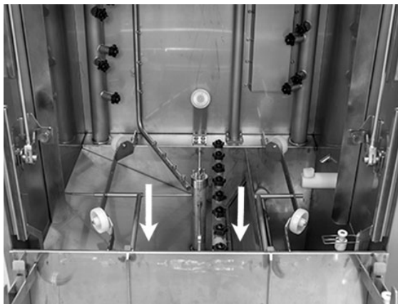
изображение 38 Очистка с нижней стороны
