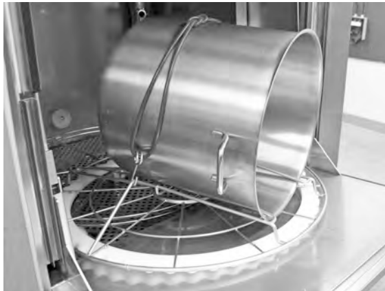
Abbildung 17 Topfkorb
