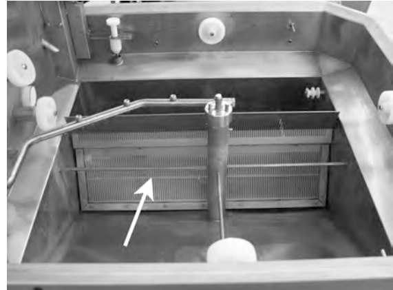
Abbildung 26 Granulatdämpfer
